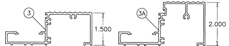
STD. SILL
